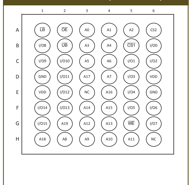
Standard SRAM Pin Configuration: 48-ball mini BGA (7.2x8.7mm)
